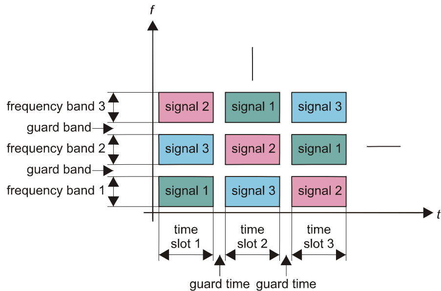
FH-CDMA
