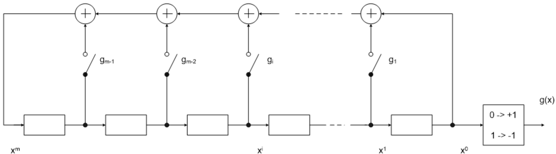
Všeobecný tvar PN generátora
